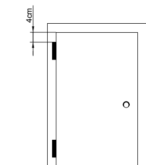
Configurazione 2 cerniere 2 hinges configuration
