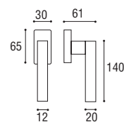
Cod. 178 CC 59 RQ Cremonese EZ Window handle EZ
