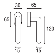
Cod. 152 CS 29 Cremonese EZ Window handle EZ
