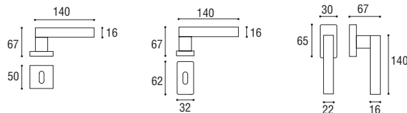
Cod. 164 CC 35 RQ Maniglia per finestra DK Window handle DK
