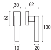
Cod. 153 CS 59 RQ Cremonese EZ Window handle EZ
