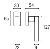
Cod. 165 CC 59 RQ Cremonese EZ Window handle EZ
