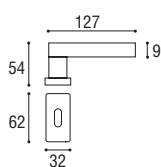
Cod. 165 CC 35 RQ Maniglia per finestra DK Window handle DK
