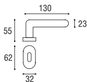
Cod. 03 CS 35 Maniglia per finestra DK Window handle DK
