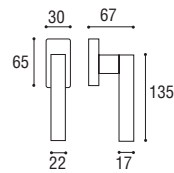
Cod. 180 CS 59 RQ Cremonese EZ Window handle EZ
