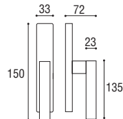
Cod. 174 CS 59 RQ Cremonese EZ Window handle EZ
