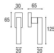
Cod. 166 CS 59 RQ Cremonese EZ Window handle EZ
