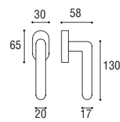
Cod. 10 CC 59 Cremonese EZ Window handle EZ
