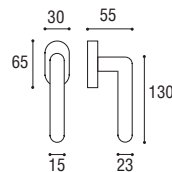
Cod. 03 CS 59 Cremonese EZ Window handle EZ
