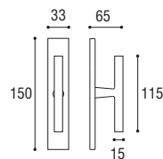
Cod. 01 CC 29 RQ Cremonese EZ Window handle EZ
