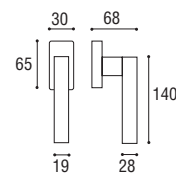
Cod. 183 CS 59 RQ Cremonese EZ Window handle EZ
