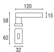
Cod. 01 CC 35 RQ Maniglia per finestra DK Window handle DK
