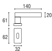
Cod. 178 CC 35 RQ Maniglia per finestra DK Window handle DK
