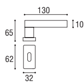
Cod. 140 CS 35 RQ Maniglia per finestra DK Window handle DK
