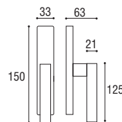
Cod. 175 CS 59 RQ Cremonese EZ Window handle EZ
