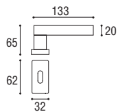
Cod. 186 CC 35 RQ Maniglia per finestra DK Window handle DK
