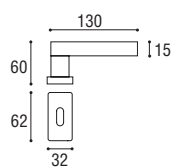
Cod. 127 CC 35 RQ Maniglia per finestra DK Window handle DK
