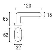
Cod. 152 CS 35 C04 Maniglia per finestra DK Window handle DK
