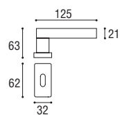
Cod. 175 CS 35 RQ Maniglia per finestra DK Window handle DK
