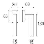
Cod. 127 CC 59 RQ Cremonese EZ Window handle EZ
