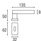
Cod. 177 CC 35 C04 RQ Maniglia per finestra DK Window handle DK
