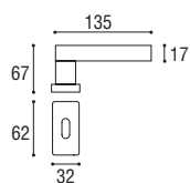
Cod. 180 CS 35 RQ Maniglia per finestra DK Window handle DK
