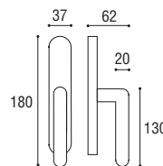
Cod. 143 OL 59 Cremonese EZ Window handle EZ
