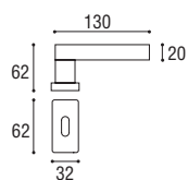
Cod. 153 CS 35 C04 RQ Maniglia per finestra DK Window handle DK
