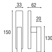
Cod. 153 CS 59 RQ Cremonese EZ Window handle EZ
