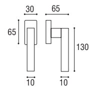
Cod. 140 CS 59 RQ Cremonese EZ Window handle EZ
