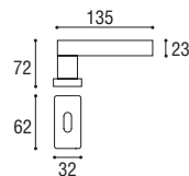
Cod. 174 CS 35 RQ Maniglia per finestra DK Window handle DK
