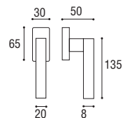
Cod. 177 CC 59 RQ Cremonese EZ Window handle EZ
