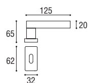
Cod. 166 CS 35 RQ Maniglia per finestra DK Window handle DK
