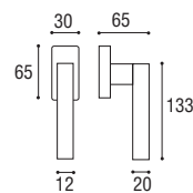
Cod. 186 CC 59 RQ Cremonese EZ Window handle EZ
