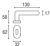
Cod. 10 CC 35 Maniglia per finestra DK Window handle DK
