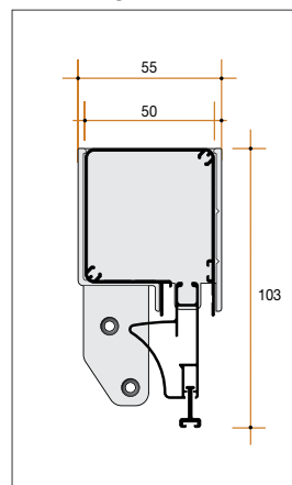
Il sistema di aggancio-sgancio CLIC-CLAK®
