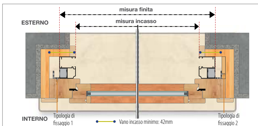
Sezione orizzontale
