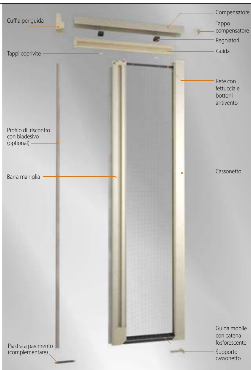
Ingombro Cassonetto e Barra maniglia.
