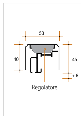
Compensatore e guida montata.
