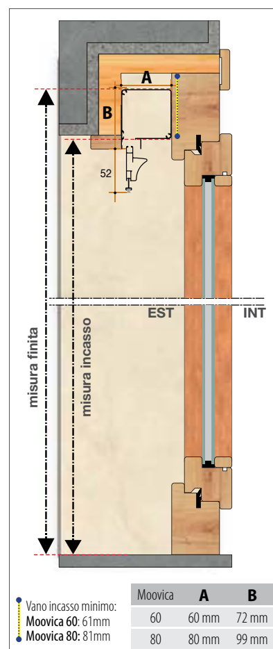
Sezione verticale
