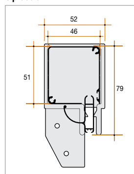
Cassonetto con barra maniglia e piastra
