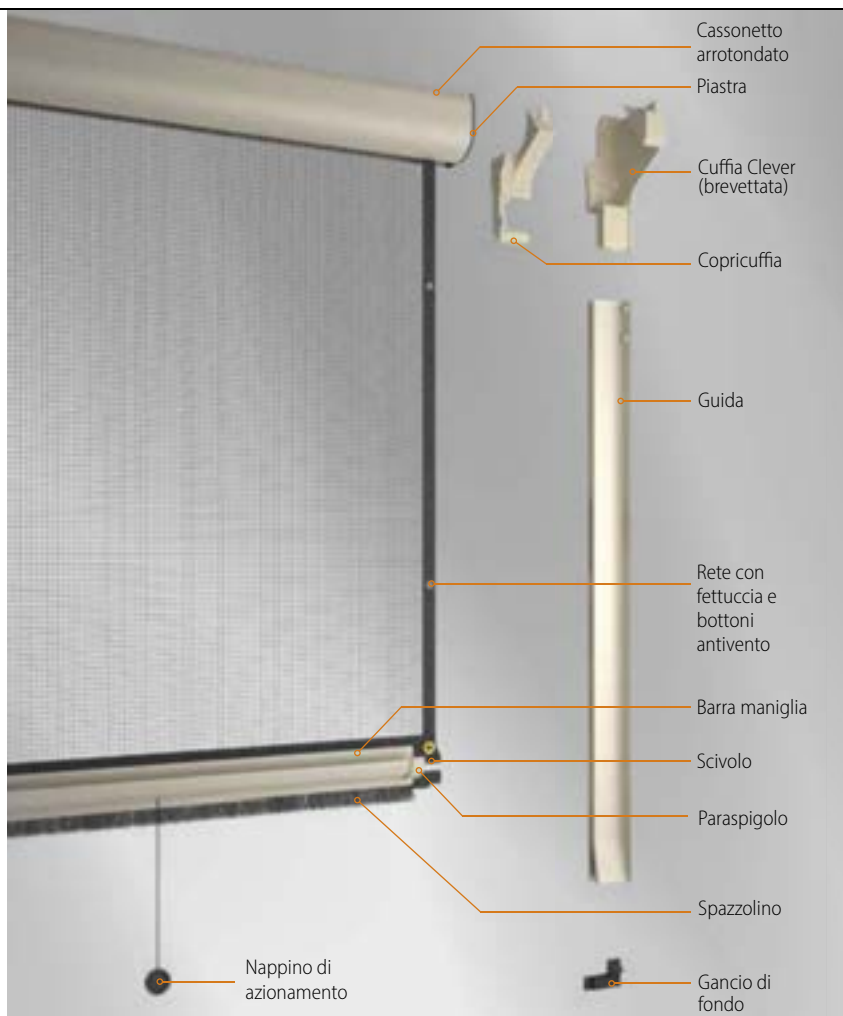
Cuffie Clever (brevetto internazionale Bettio)
