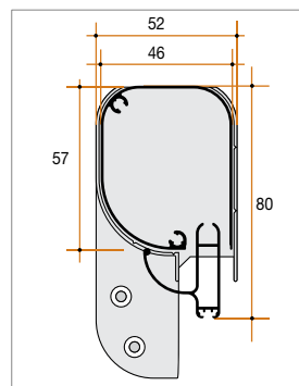
La guida telescopica (optional)
