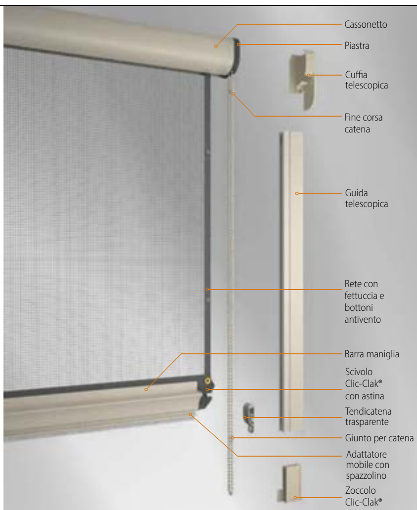
La guida telescopica
