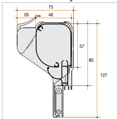
Cassonetto con barra maniglia e cuffia Clever
