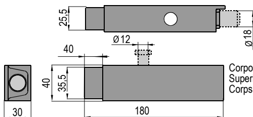
Corpo centrale Central body Corps centrale
