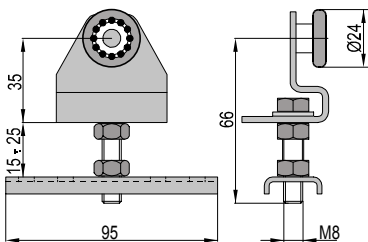
Fix trolley with 1 wheel. Chariot fixe à 1 roulement.
