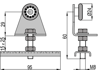
Fix trolley with 1 wheel. Chariot fixe à 1 roulement.
