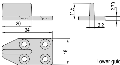
Lower guide in plastic. Guide inférieur en plastique.
