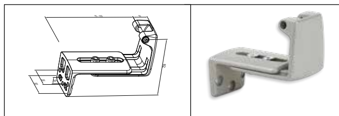
Staffa vasistas regolabile a "Z" in pressofusione GRIGIO cod. 41709Z NERO cod. 41710A BIANCO cod. 41711B
