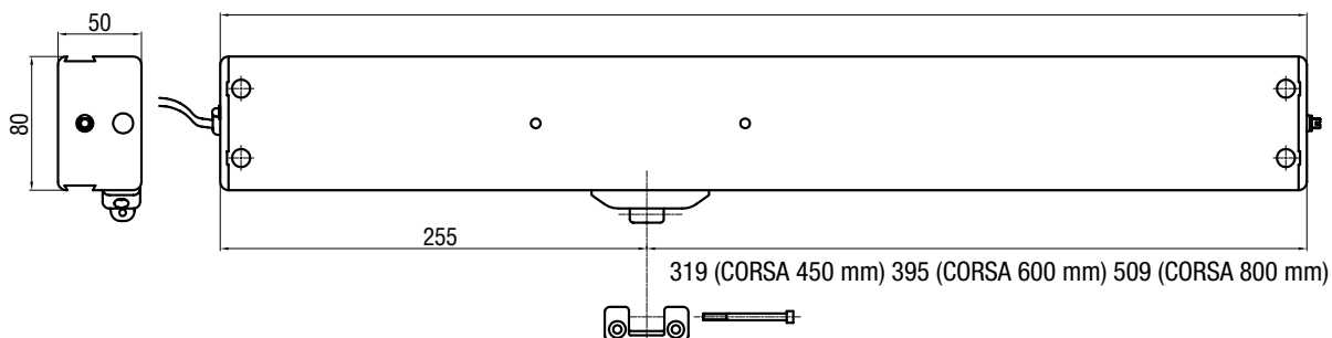
Dimensioni attuatore
