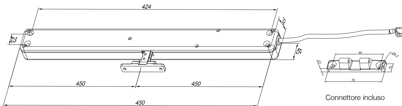
Dimensioni attuatore
