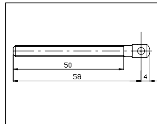
Puntale catena per applicazioni special(es. serramenti in legno, PVC) cod. 81222C
