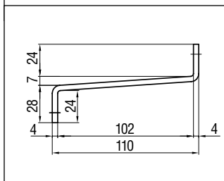
Staffa per vasistas in alluminio cod. 40157I per impianti EFC e serramenti pesanti
