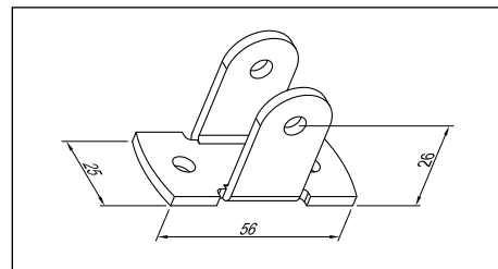
Connettore frontale in acciaio cod. 41927I
