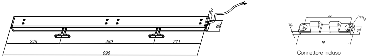
Dimensioni Twin Vega
