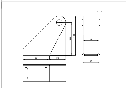
Staffa anteriore in alluminio cod. 356960 Consente il fissaggio del cilindro al telaio fisso del serramento e la rotazione, in fase di apertura, del cilindro stesso. La staffa è collegata al cilindro tramite i raccordi/supporti.
