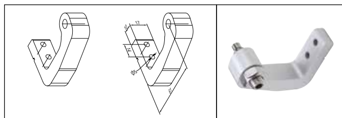
Staffe oscillanti a "C" (da ordinare separatamente): ALLUMINIO ANODIZZATO cod. 41197Z NERO RAL 9005 cod. 41198A BIANCO RAL 9010 cod. 41199B
