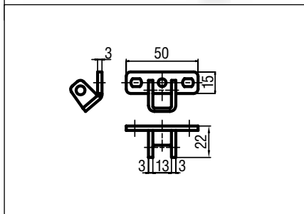
Connettore in acciaio zincato cilindro-serramento per ventilazione cod. 40252G
