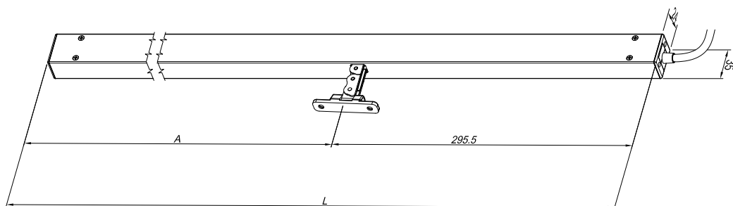
Dimensioni attuatore
