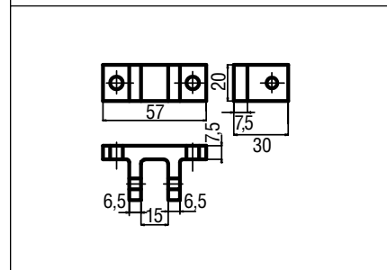
Connettore in alluminio cilindro-serramento cod. 35697P
