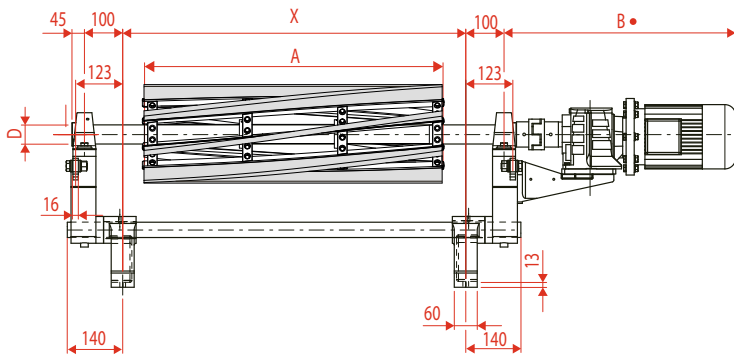
UST: Unità Spazzolante Normale con motoriduttore a flangia e regolazione a tirante / Standard Brushing Unit with flange mounted gearbox and pulling rods
