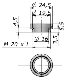
Bussola per installazione maniglia senza rosetta Bush for latch lock handle without washer
