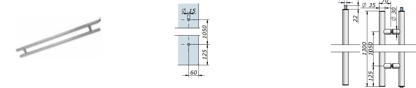
Maniglione tubolare con chiave su un lato Tubular handle with lock on one side
