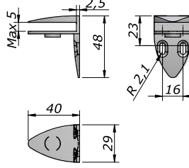
Cerniera sagomata senza tacca per spessore max 5 mm Oval hinge without cutout for maximum 5 mm thickness
