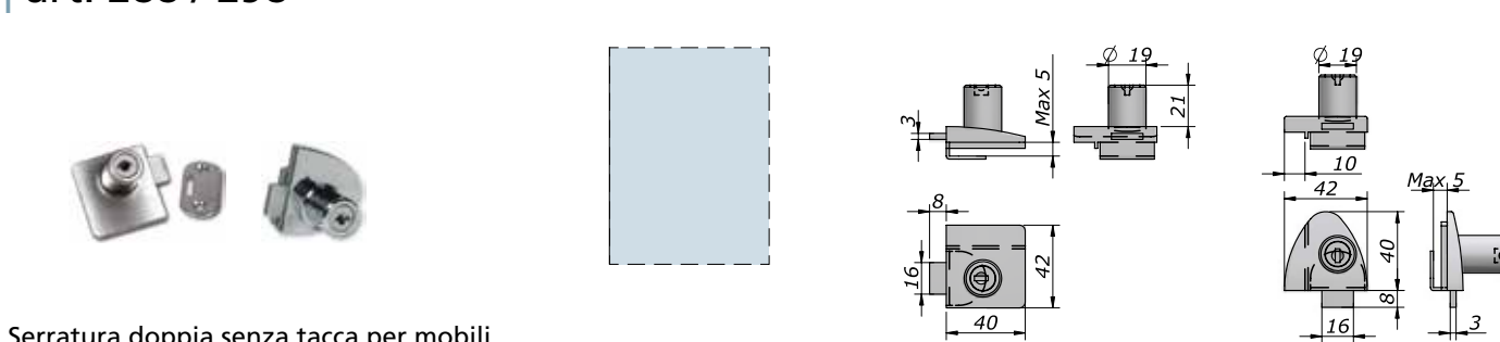
Serratura doppia senza tacca per mobili Double furniture lock without cut-out
