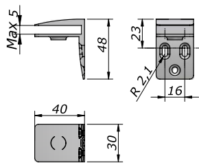
Cerniera quadrata senza tacca per spessore max 5 mm Square hinge without cutout for maximum 5 mm thickness
