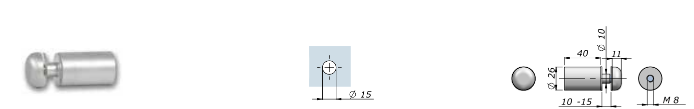
Distanziale con borchia Spacer with cap
