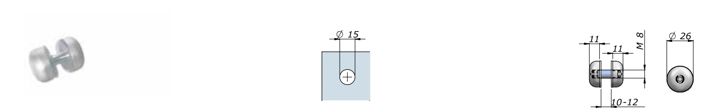
Doppia borchia Double boss
