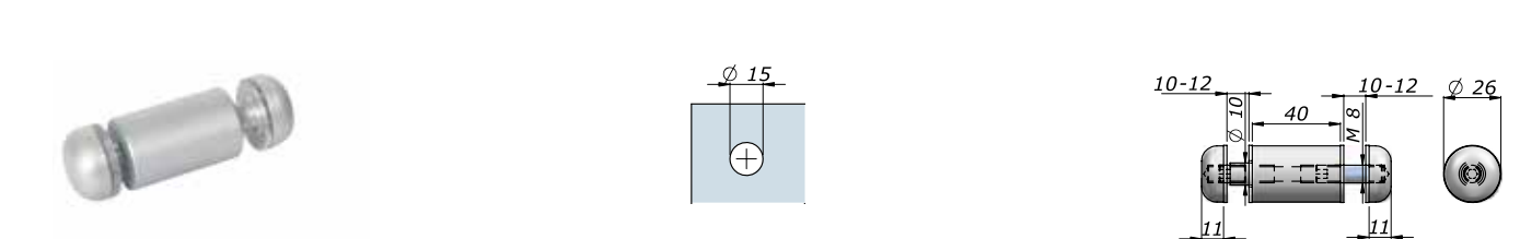
Distanziale con borchia doppia Spacer with double cap
